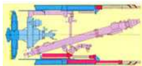
子機離脱状態図
