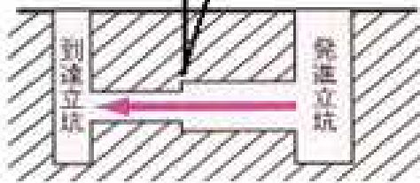
親子シールド概念図
