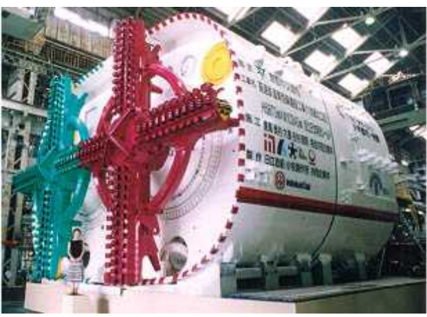
矩形シールド(地下鉄向け) H6.87m × W10.24m
