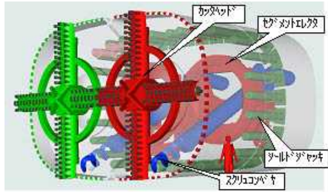
揺動式カッタヘッド
