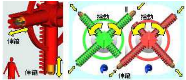
揺動式カッタヘッド
