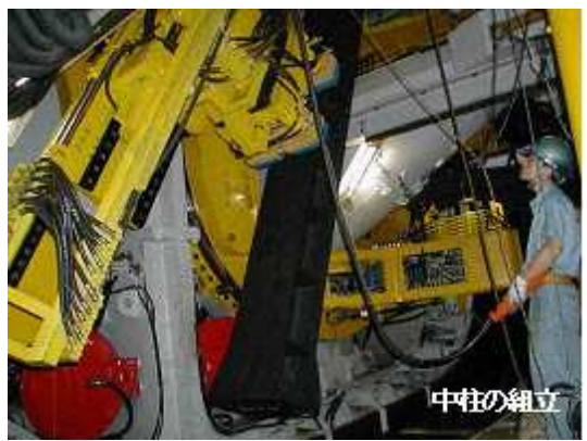
矩形シールド H4.3m × W.4.9m
